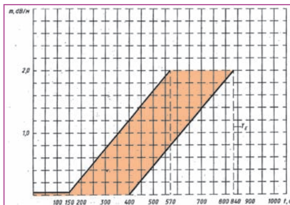
Рис. 2.2. Зависимость оптической плотности среды от времени при тестовом пожаре ТП-2 (горение древесины)
