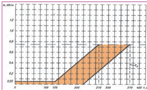
Рис. 2.1. Зависимость оптической плотности среды от времени при тестовом пожаре ТП-1 (тление древесины)
