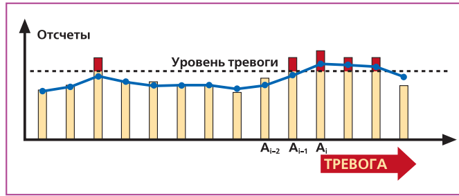
Рис. 5.1. Вычисление огibaющей
