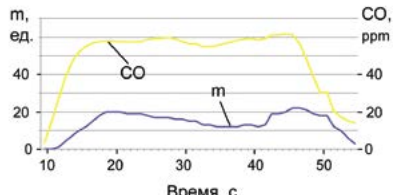
Рис. 14. Оптическая плотность и концентрация CO при тлении хлопкового фитиля на входе трубки
