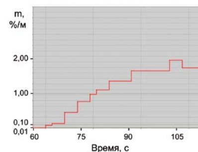
Рис. 8. Оптическая плотность дыма при тлении хлопкового фитиля с повышенной мощностью аспиратора
