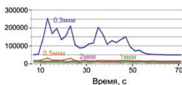
Рис. 18. Нормированная концентрация частиц дыма различного размера при тлении хлопковой нитки на входе трубки
