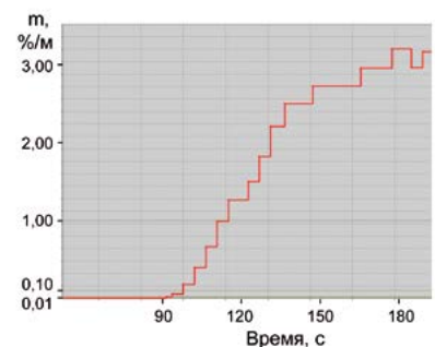
Рис. 7. Оптическая плотность дыма при тлении хлопкового фитиля
