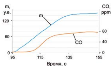
Рис. 12. Оптическая плотность и концентрация СО при тлении хлопкового фитиля в трубке
