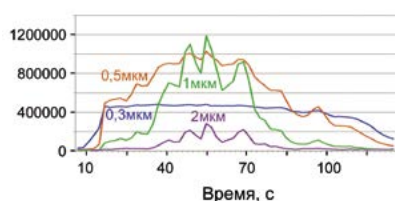
Рис. 16. Нормированная концентрация частиц дыма различного размера при тлении хлопковой нитки в коробке
