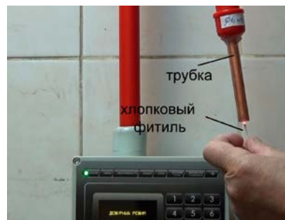
Рис. 5. Тление хлопкового фитиля в трубке \varnothing 10 мм
