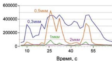
Рис. 17. Нормированная концентрация частиц дыма различного размера при тлении хлопковой фитили в трубке
