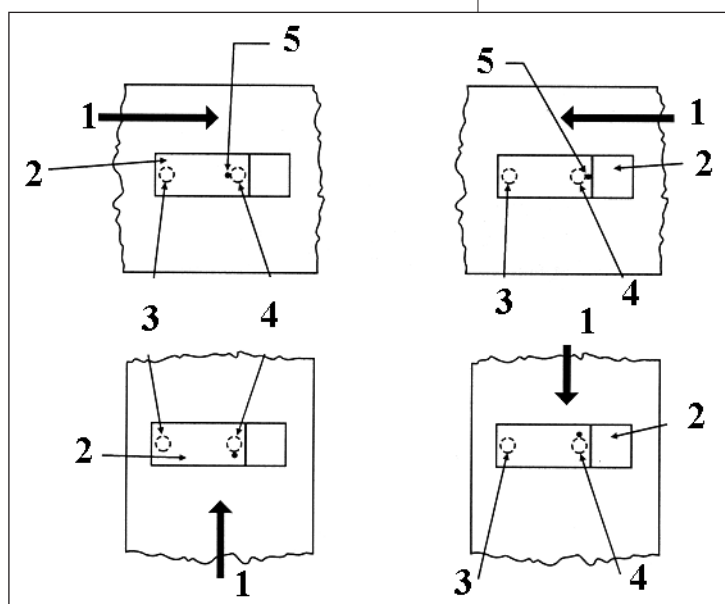
Рис. 5 Различные способы установки корпуса DH400
