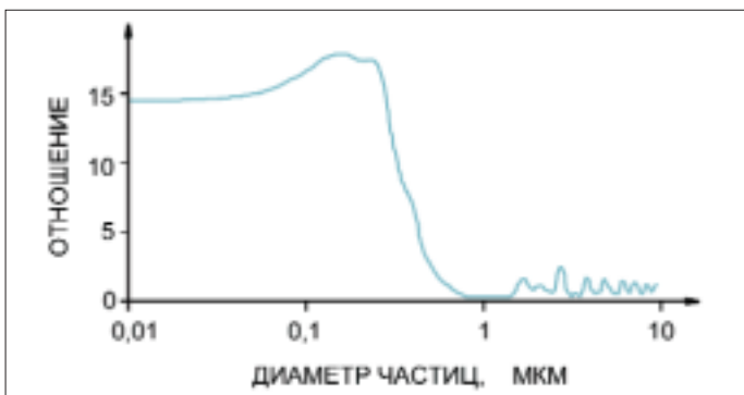
Рис. 4. Отношение рассеяния синего света к инфракрасному в зависимости от размера частиц
