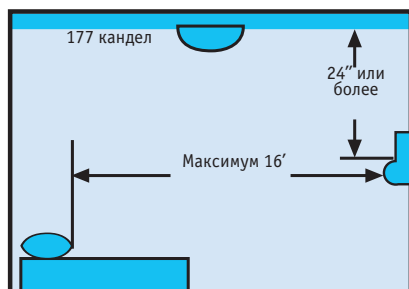
Рис. 8. Расположение световых оповещателей в спальном помещении
