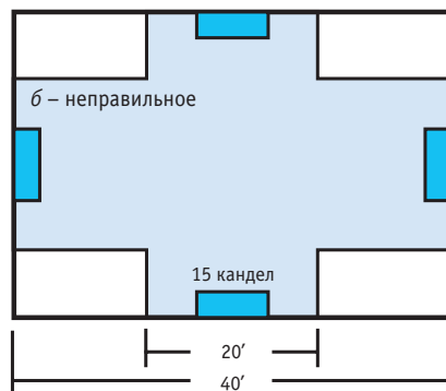
Рис. 7. Расположение настенных световых оповещателей в обычном помещении
