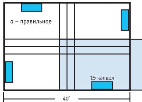
Рис. 6. Потолочная установка. Распределение в нижней полусфере
