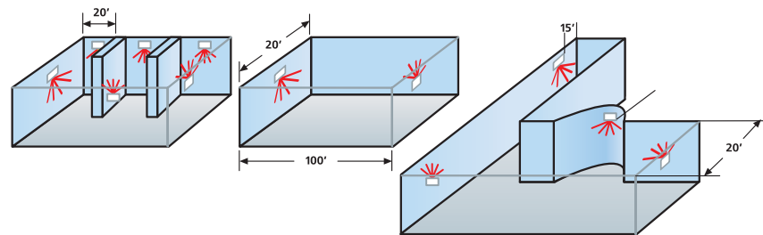
Рис. 9. Расположение световых оповещателей в коридорах
