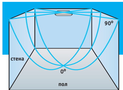
Рис. 6. Потолочная установка. Распределение в нижней полусфере
