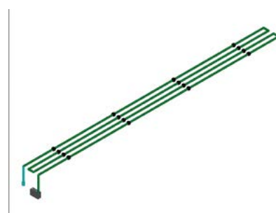
Рис. 1. Конфигурация трубы аспирационного извещателя. Точками обозначены отверстия в трубе
