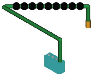
Рис. 5. Конфигурация трубы аспирационного извещателя. Точками обозначены отверстия в трубке
