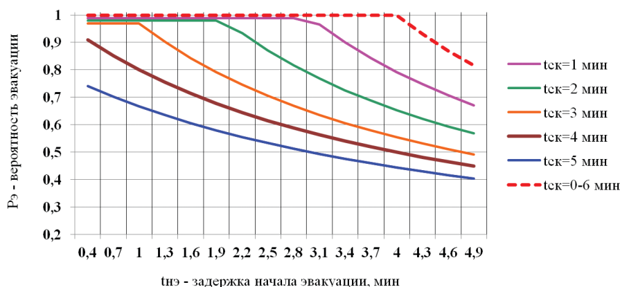
Рис. 4. Зависимость вероятности эвакуации людей P_{э} от времени задержки начала эвакуации и времени скопления для t_{об} = 20 мин, t_{эв} = 12 мин
