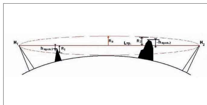
Рис. 4. Определение значений просвета h_{преп.1} , h_{преп.2} – расстояние от высшей точки препятствия до линии прямой видимости (м)
