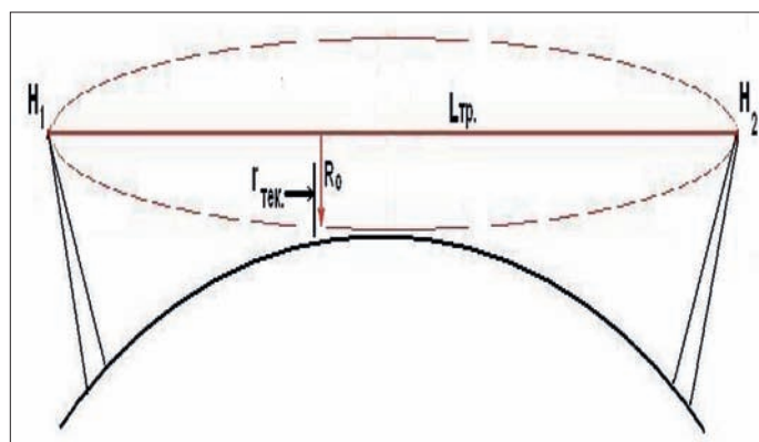
Рис. 3. Определение зоны Френеля
