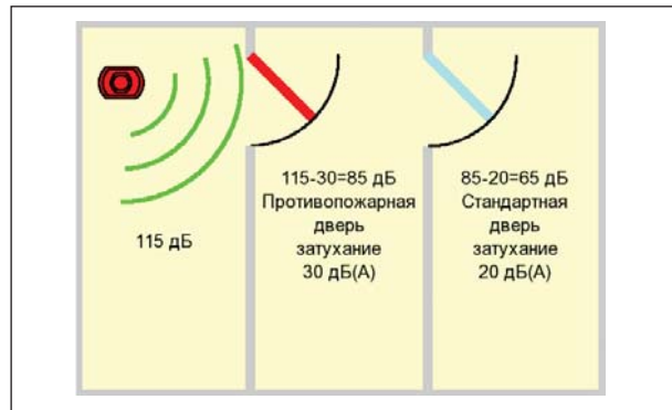
Рис. 2 Снижение уровня сигнала при наличии дверей
