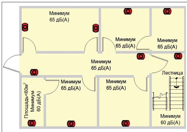
Рис. 10 Минимальные уровни сигналов оповещения по европейским нормам
