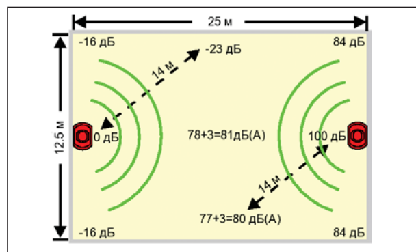
Рис. 3 Уровни сигнала оповещения в различных частях помещения
