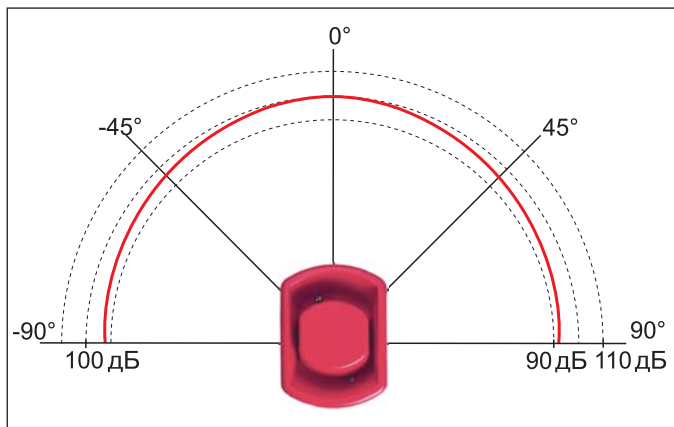
Рис. 4 Диаграмма направленности оповещателя серии ЕМА
